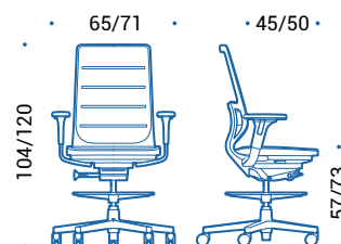
SFA.256 | sgabello girevole, regolabile in altezza, meccanismo di oscillazione syncro auto-fit, supporto lombare regolabile
